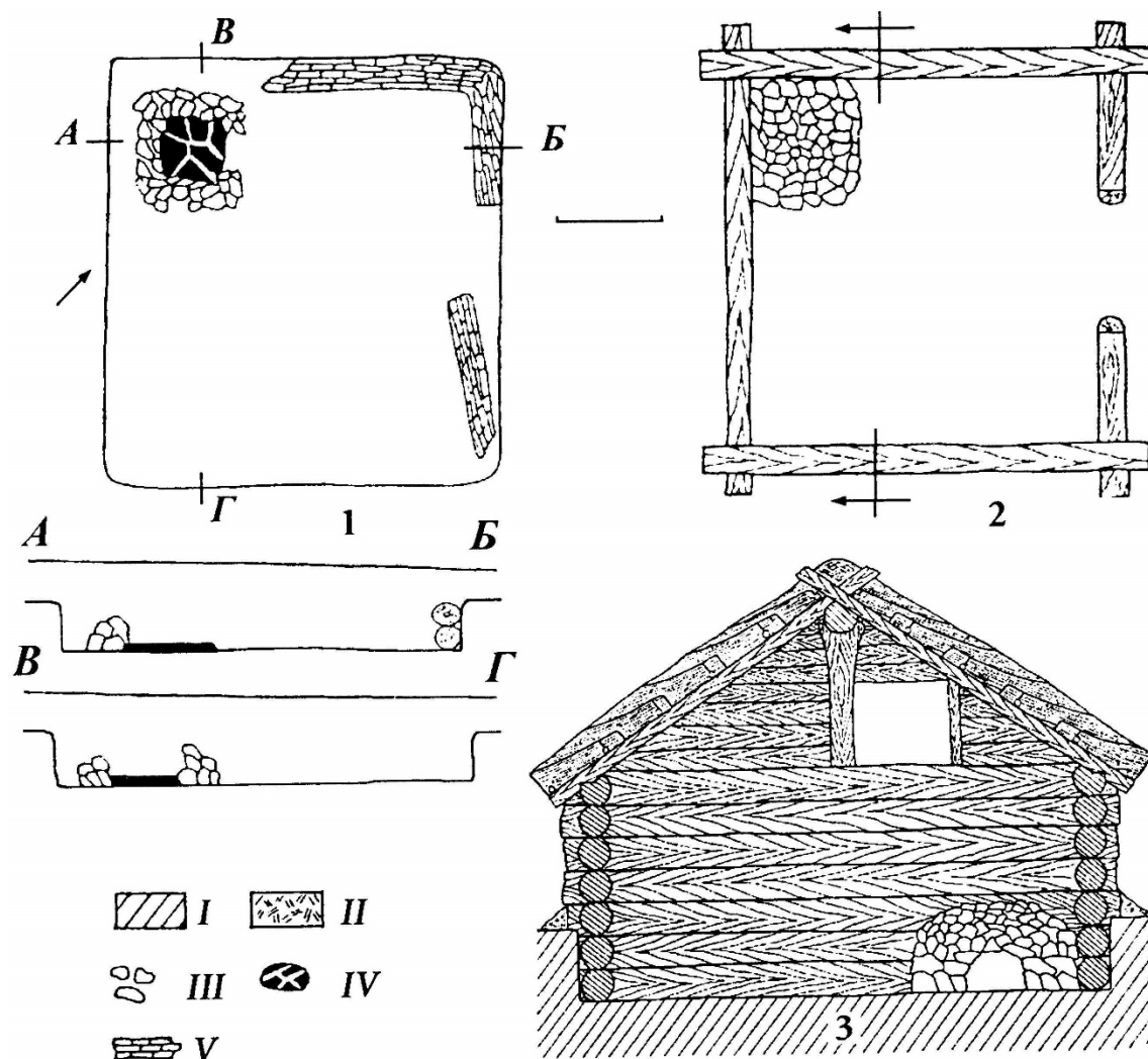
Рис. 2. Реконструкция срубной полуземлянки V-VII вв. (По О. М. Приходнюку): 1 – полевой план (I – материк, II – насыпной грунт; III – камень; IV – черень; V – обугленное дерево); 2 – реконструкция полевого плана полуземлянки без перекрытия; 3 – реконструкция полуземлянки
